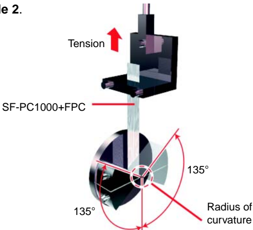
Fig. 4 MIT flexural endurance test
