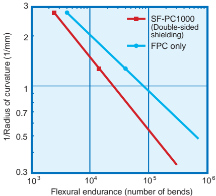
Fig. 5 MIT flexural endurance characteristics
